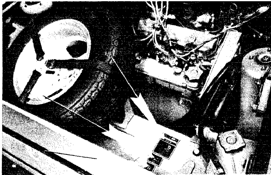
Posizione stampigliatura e targhetta per l'identificazione della vettura. Position de l'estampillage et de la plaquette pour l'identification de la voiture. Position of the stamping and plate for the identification of the car. Position der Einstanztg und des Schildes mit den Kenndaten des Wagens.
